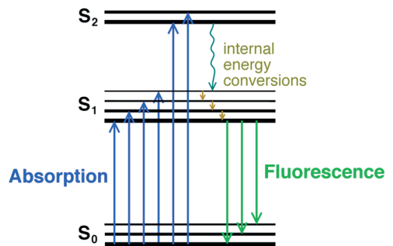
Figura 1. Esquema de los diferentes niveles de energía S de los electrones como consecuencia de la absorción de la luz solar y la emisión de fluorescencia. S 0 es el estado basal o fundamental. S 1 y S 2 son estados excitados.
