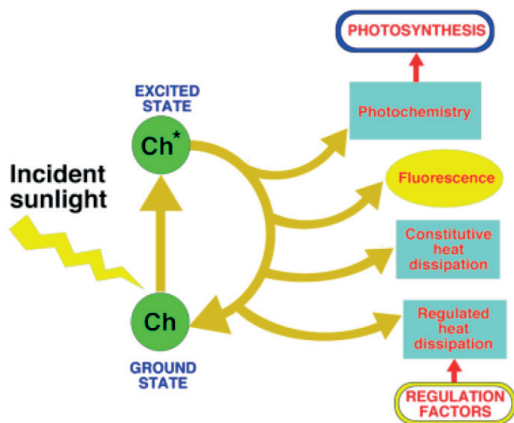
Figura 2. Esquema de la energía lumínica capturada por las moléculas de clorofila y los diferentes mecanismos de disipación de energía.
