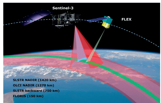
Figura 4. Composición artística del tándem Sentinel-3 y FLEX (ESA, 2013).
