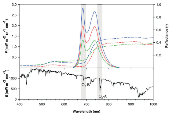
Figura 3. Señal simulada con FluorSAIL3.0 de fluorescencia (arriba) de tres vegetales diferentes junto a la curva de reflectividad (en líneas discontinuas). Abajo, irradiancia solar (Meroni et al. , 2010).
