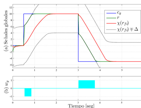
Figura 7: Topología global: (a) Consigna global, referencia global y media de las referencias locales, junto con la banda o región permitida. (b) Acción discontinua.
