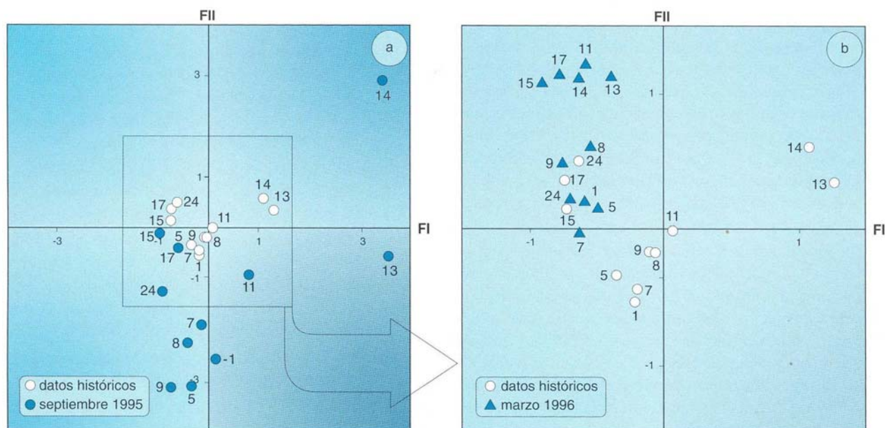
Figura 6. Representación de la disposición de las distintas estaciones de muestreo en el plano definido por las variables FI y FII, para situaciones diferentes. En ambos casos se representa la ubicación de las estaciones según del ACP de los datos históricos. En (A) se añade la representación de las estaciones según los datos obtenidos en septiembre de 1995. En (B) se superponen los datos correspondientes a la campaña de marzo de 1996.
