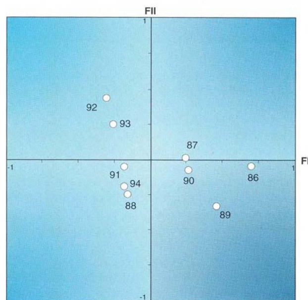
Figura 4. Representación de los valores medios anuales de FI y FII agrupados por años naturales y promediados. Tan sólo se representan los años 1986-1994, por ser los que presentan una mayor regularidad en el muestreo
