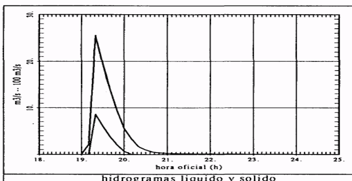
Figura 18 Hidrograma real y sedimento grama supuesto del 12-08-93.
