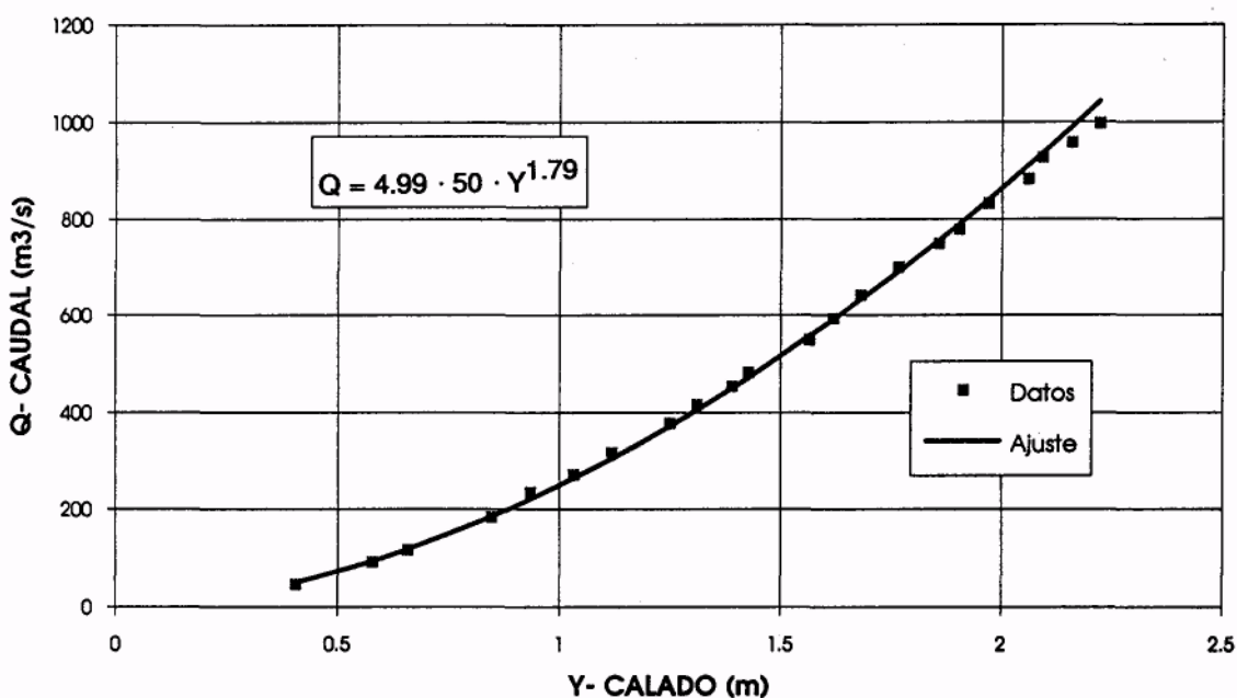
Figura 9 Ajuste de la curva de vertido en la estación de aforos del prototipo.
